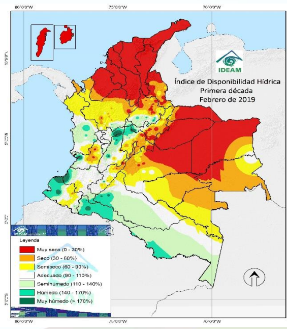
Figura 2. Índice de disponibilidad hídrica de la tercera década de enero y primera década de febrero de 2019
