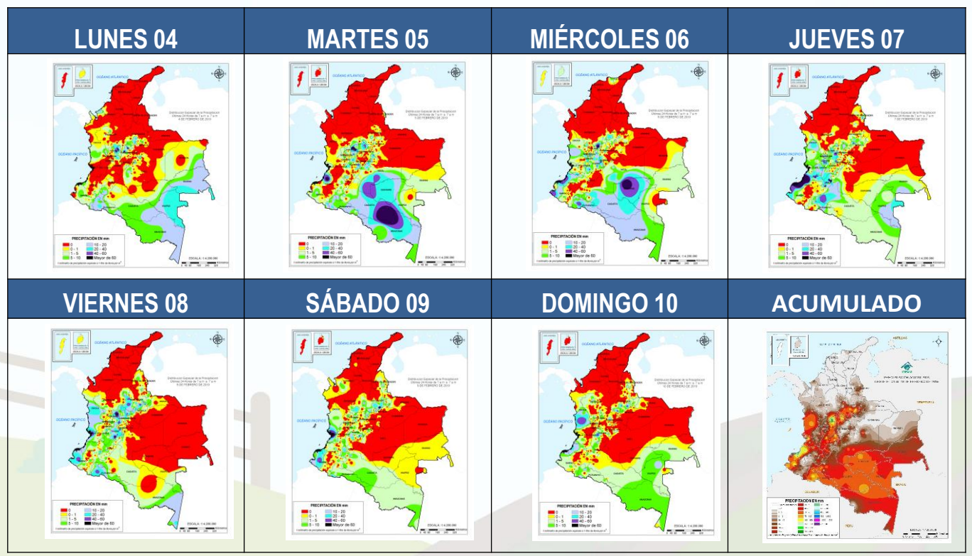
Figura 1. Precipitación diaria acumulada desde el lunes 04 al domingo 10 de febrero de 2019. Fuente: Grupo de datos OSPA - IDEAM
