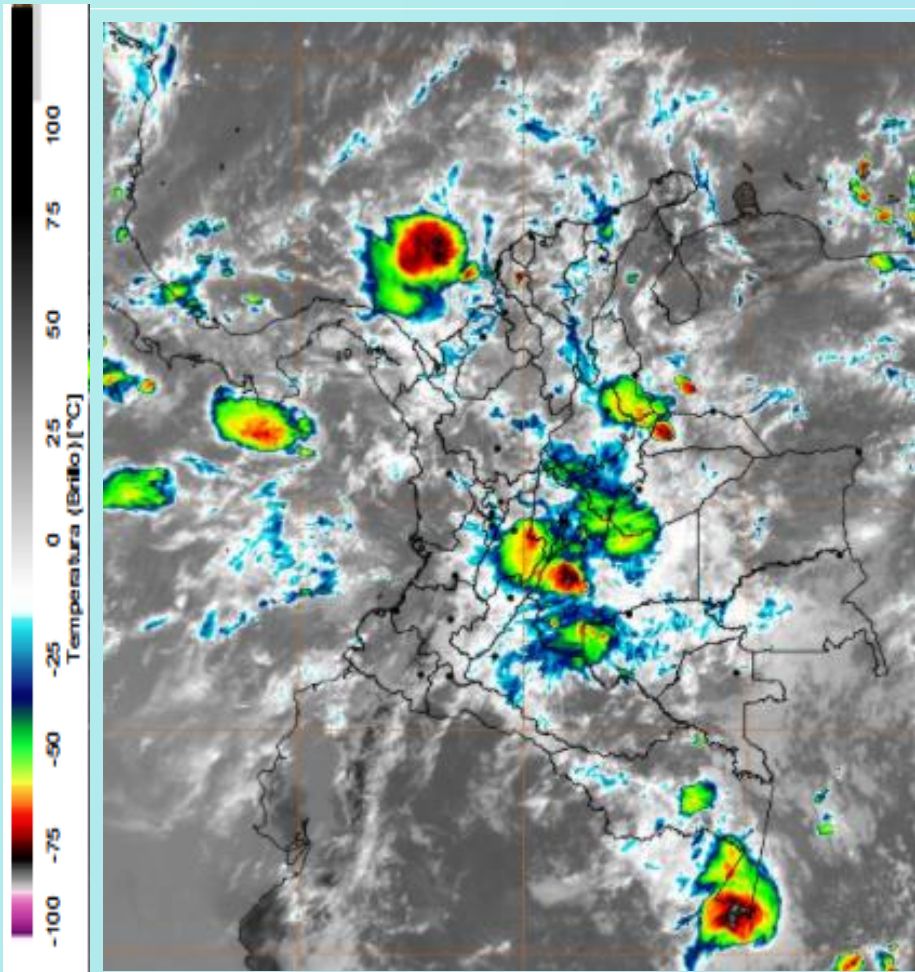
Imagen GOES East Canal Infrarrojo, 17 de agosto de 2020. Hora 11:40 HLC. Fuente: IDEAM-GOES 16
