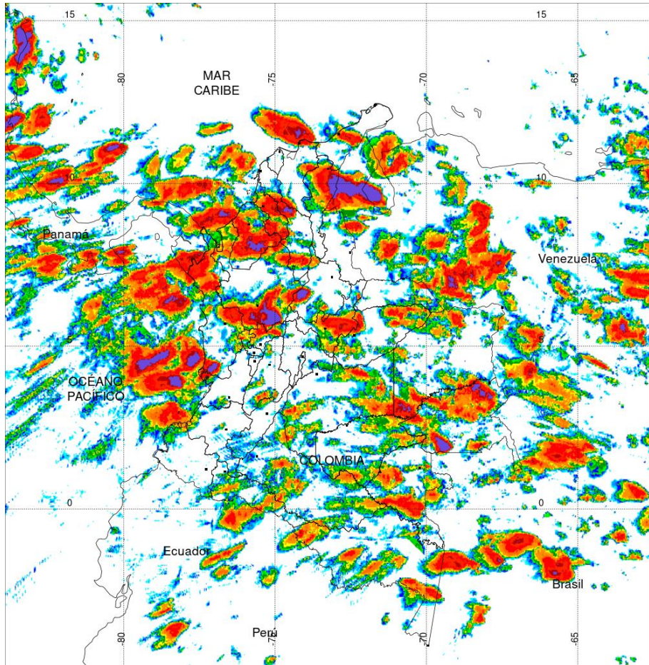
PRECIPITACIÓN TOTAL ACUMULADA POR ESTIMACIÓN SATELITAL (GOES-16) AUG 16 DE 2020 (7:00) - AUG 17 DE 2020 (7:00)
