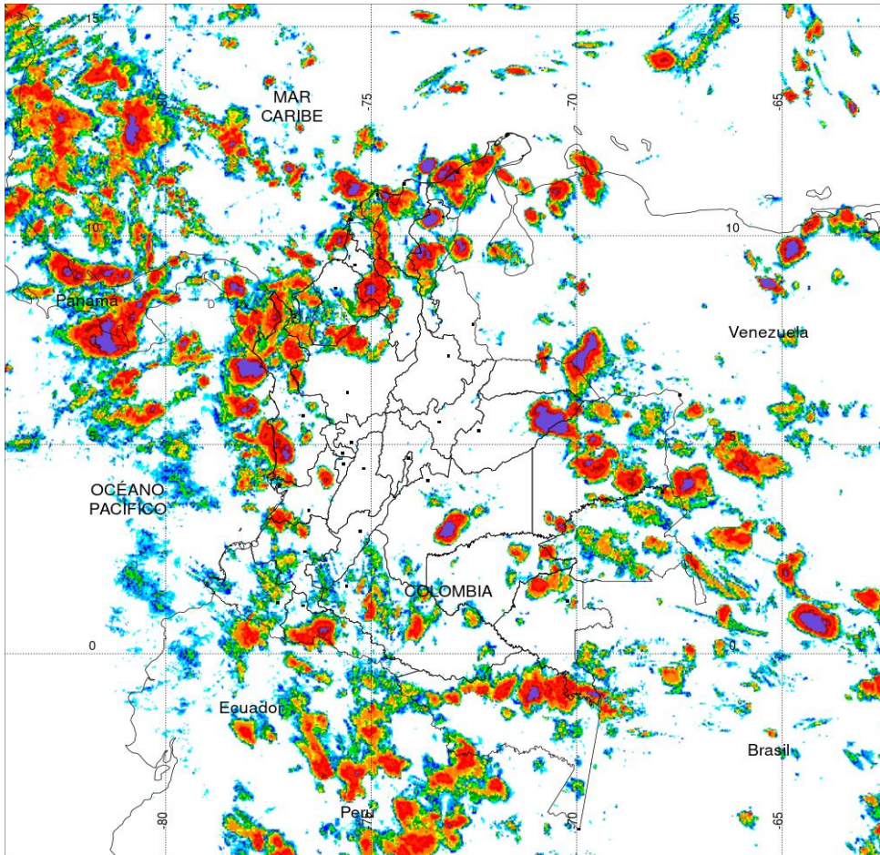
PRECIPITACIÓN TOTAL ACUMULADA POR ESTIMACIÓN SATELITAL (GOES-16) SEP 13 DE 2020 (7:00) - SEP 14 DE 2020 (7:00)
