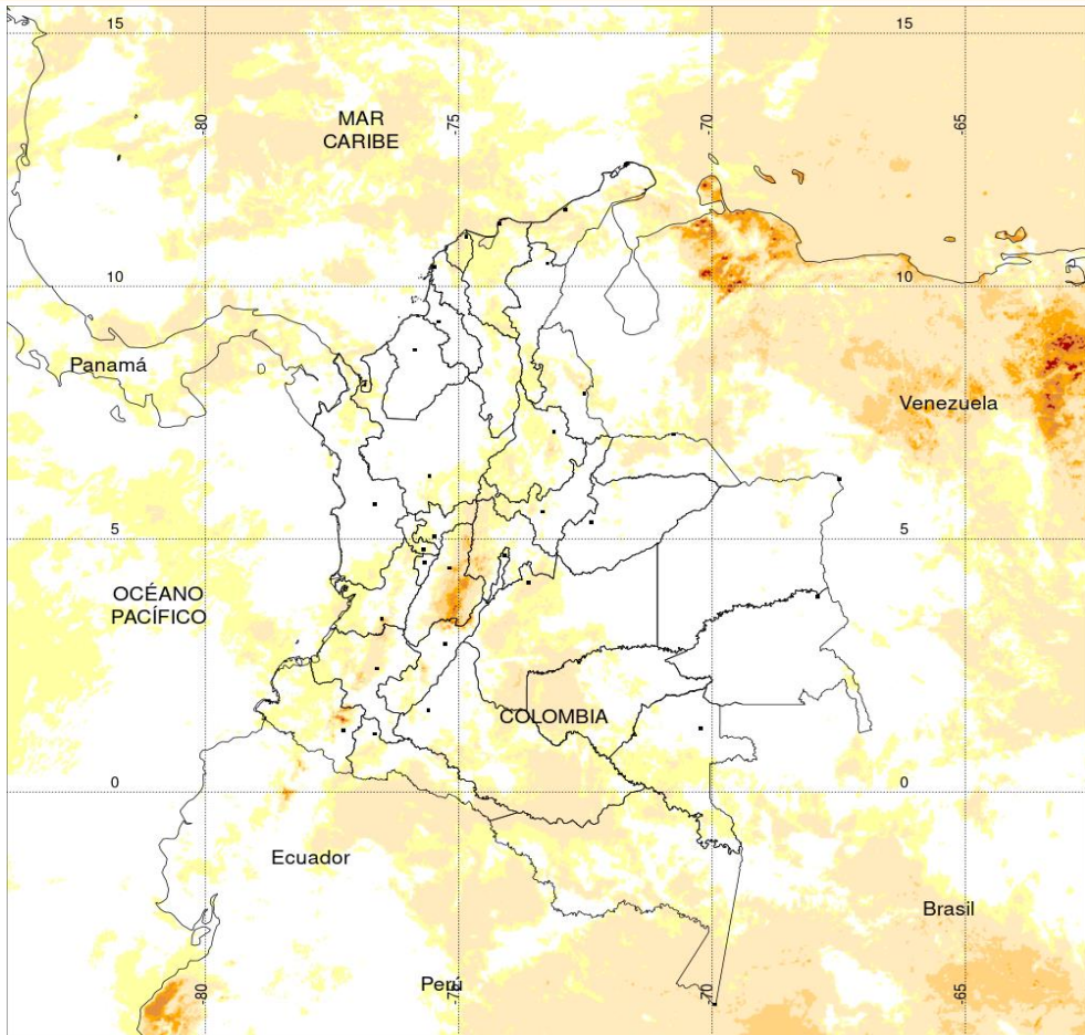
TEMPERATURA SUPERFICIAL MÁXIMA POR ESTIMACIÓN SATELITAL (GOES-16) ( 2020-09-14 09:00:00 a 2020-09-14 09:10:00 )
