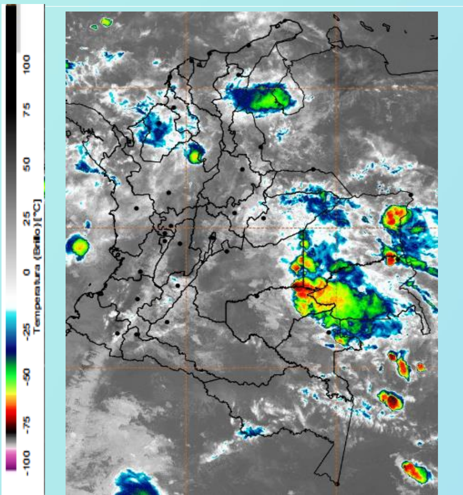
Imagen GOES East Canal Infrarrojo, 14 de septiembre de 2020. Hora 09:40 HLC. Fuente: IDEAM-GOES 16
