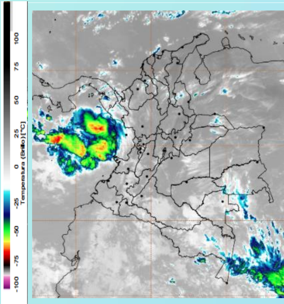
Imagen GOES East Canal Infrarrojo, 14 de enero de 2021. Hora 08:40 HLC. Fuente: IDEAM-GOES 16
