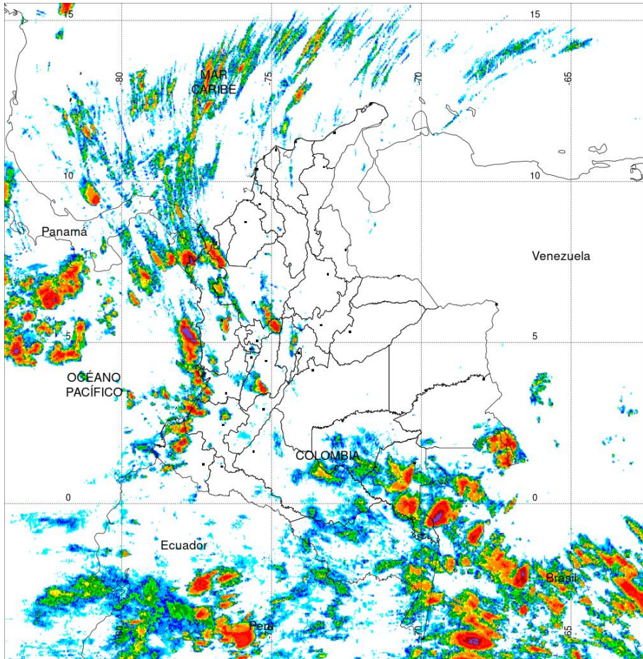
PRECIPITACIÓN TOTAL ACUMULADA POR ESTIMACIÓN SATELITAL (GOES-16) JAN 13 DE 2021 (7:00) - JAN 14 DE 2021 (7:00)
