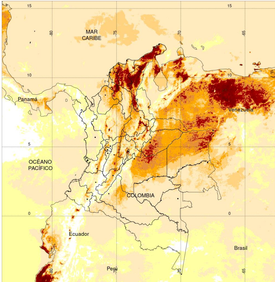
TEMPERATURA SUPERFICIAL MÁXIMA POR ESTIMACIÓN SATELITAL (GOES-16) ( 2021-01-13 09:00:00 a 2021-01-13 18:30:00 )
