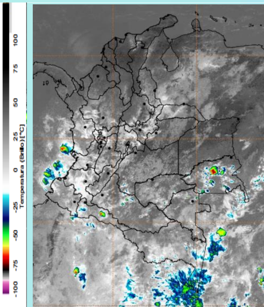
Imagen GOES East Canal Infrarrojo, 04 de febrero de 2022 - Hora 11:50 HLC. Fuente: https://rammb-slider.cira.colostate.edu/
