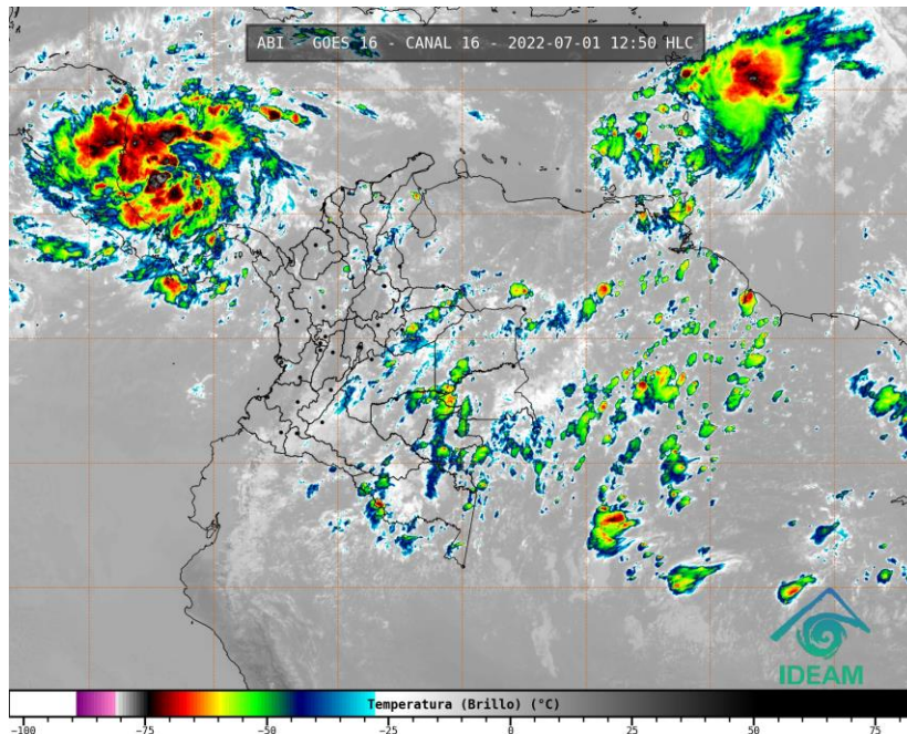
Gráfica 1. Imagen satelital canal infrarrojo GOES -16, del 01 de julio de 2022. Hora 12:50 HLC.
