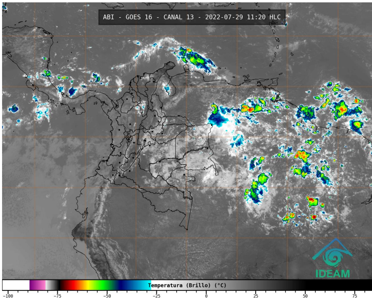
Gráfica 1. Imagen satelital canal infrarrojo GOES - 16, del 29 de julio de 2022. Hora 11:20 HLC.
