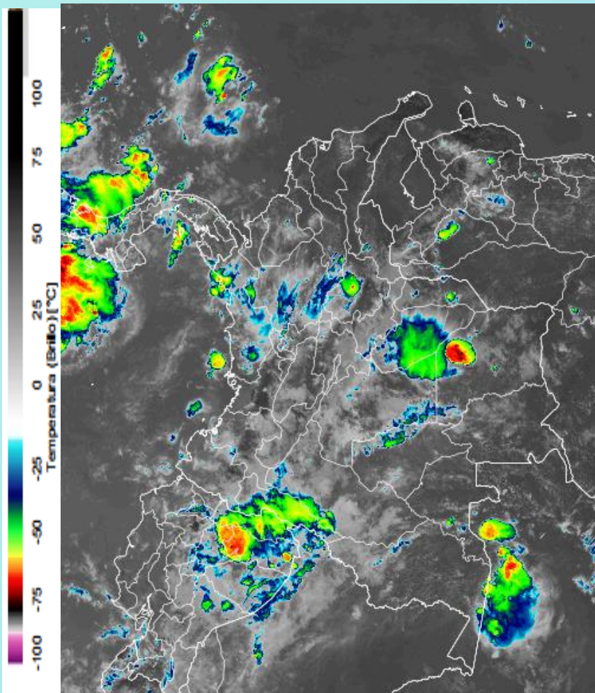
Imagen GOES East Canal Infrarrojo, 10 de octubre de 2023 - Hora 12:00 HLC. Fuente: GOES 16
