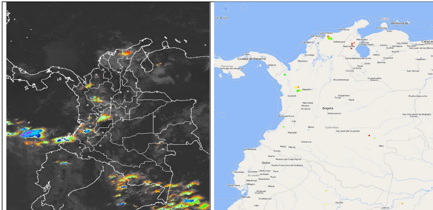
Izquierda: Imagen satelital GOES-13. Hora 4:45 p.m. HLC. Viernes 01 de enero de 2016. Derecha: Sistema de monitoreo de tormentas eléctricas en Colombia. Los puntos rojos indican las tormentas eléctricas más recientes y los verdes las más antiguas (actividad de las últimas tres horas).
