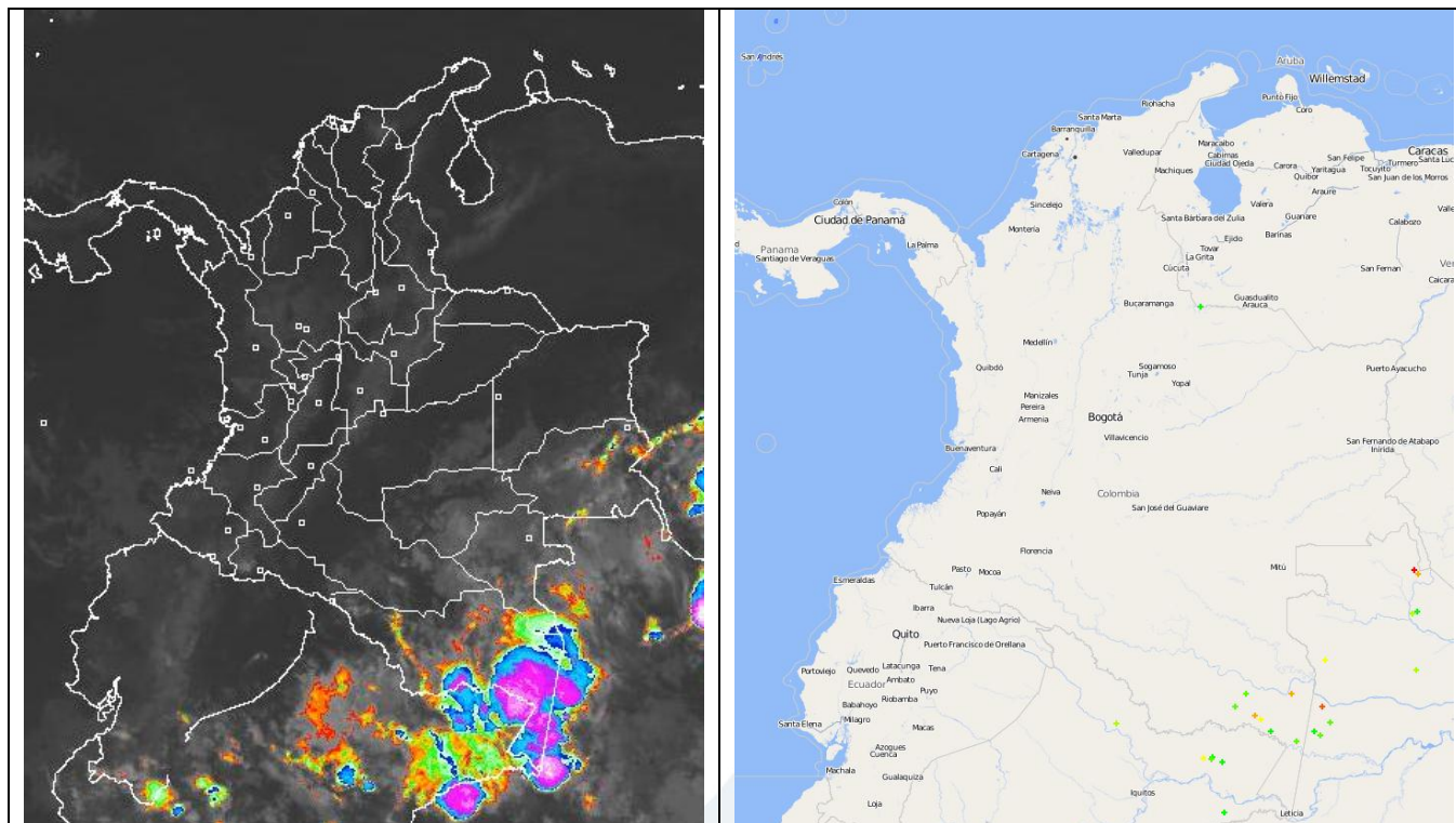
Izquierda: imagen satelital GOES-13. Hora 12:15 a.m. HLC. Martes 2 de febrero de 2016. Derecha: sistema de monitoreo de tormentas eléctricas en Colombia. Los puntos rojos indican las tormentas eléctricas más recientes y los verdes las más antiguas (actividad de la última hora).
