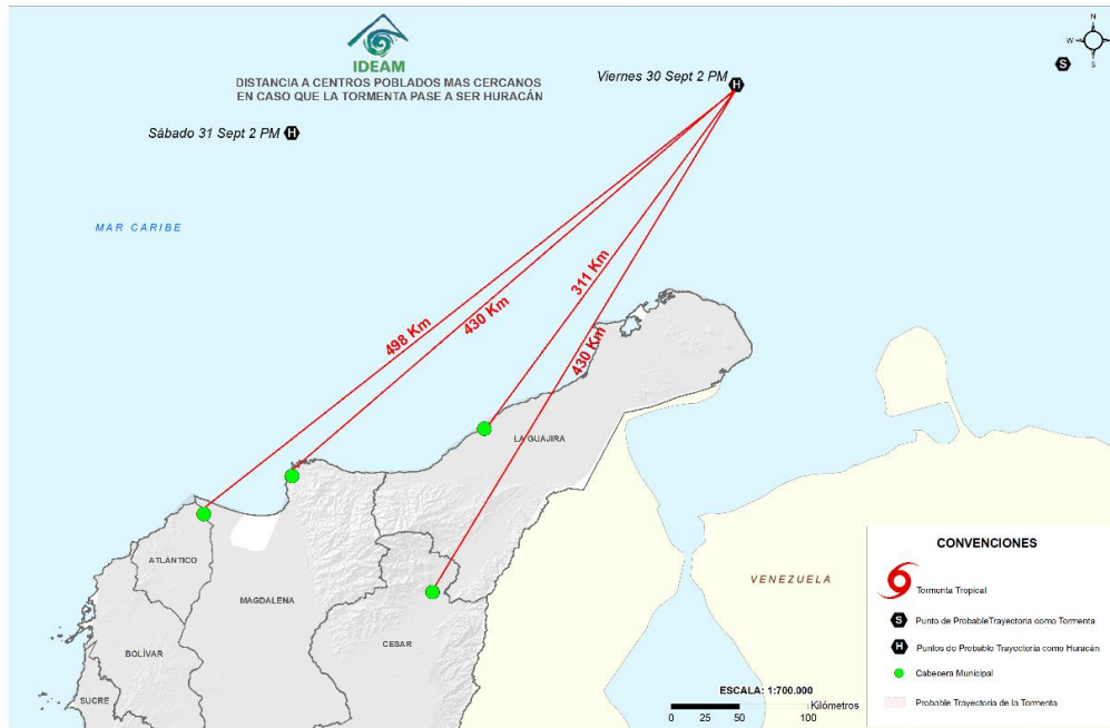
Figura 2. Pronóstico de la distancia del ciclón tropical “MATTHEW” el día viernes a las 2:00 p.m. a algunas ciudades de la región Caribe. Fuente de datos: NHC/NOAA. Elaboración propia.
