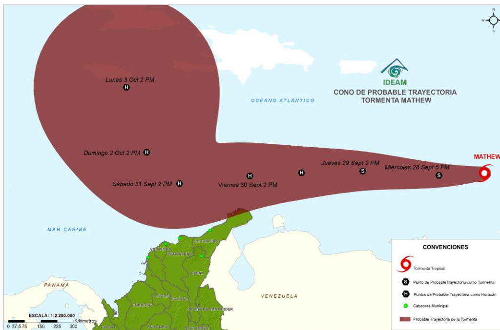
Figura 1. Pronóstico de la probable trayectoria del ciclón tropical “MATTHEW”. Fuente de datos: NHC/NOAA. Elaboración propia.
