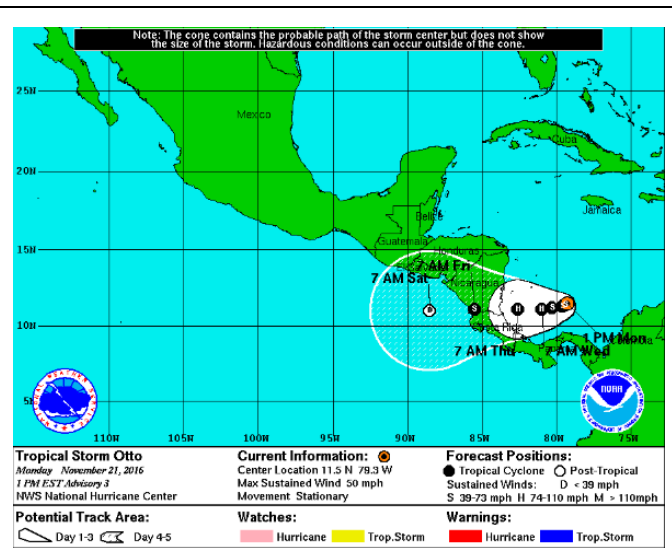
Figura 2. Trayectoria probable de la tormenta Tropical OTTO de acuerdo con el NHC.
