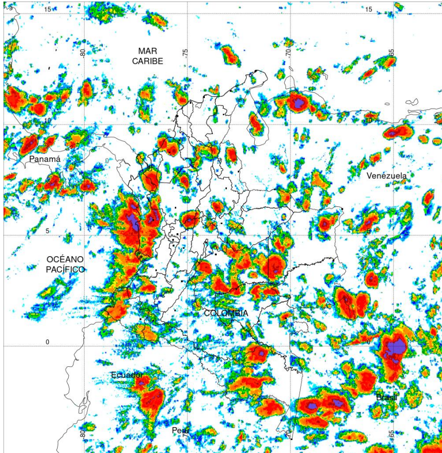
PRECIPITACIÓN TOTAL ACUMULADA POR ESTIMACIÓN SATELITAL (GOES-16) OCT 20 DE 2019 (7:00) - OCT 21 DE 2019 (7:00)
