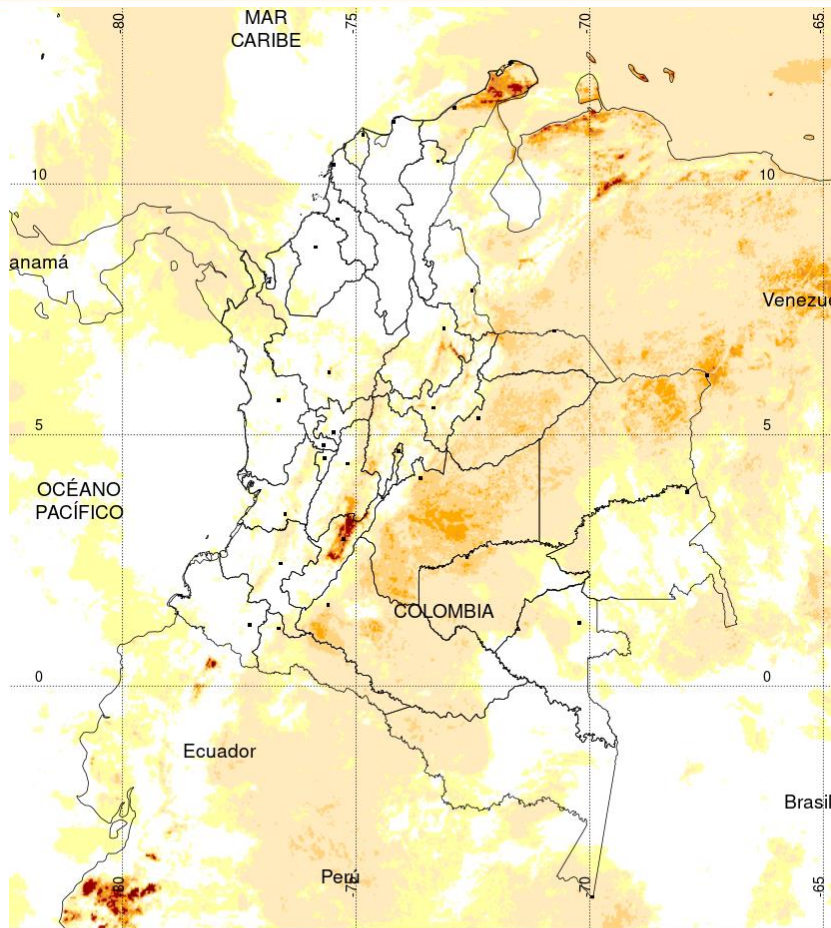
TEMPERATURA SUPERFICIAL MÁXIMA POR ESTIMACIÓN SATELITAL (GOES-16) ( 2019-10-21 09:00:00 a 2019-10-21 11:30:00 )
