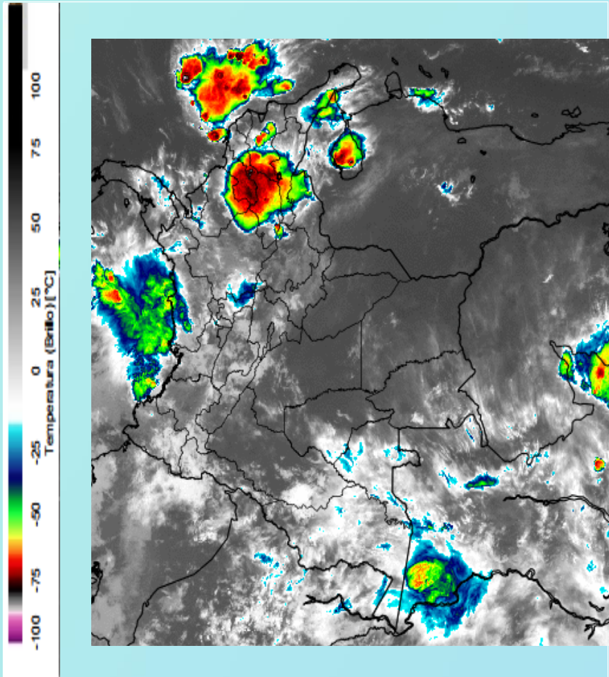
Imagen GOES East Canal Infrarrojo 21 de octubre de 2019. Hora 7:00 HLC. Fuente: IDEAM-GOES 16
