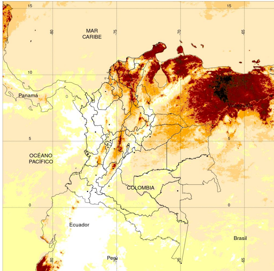
TEMPERATURA SUPERFICIAL MÁXIMA POR ESTIMACIÓN SATELITAL (GOES-16) (2020-05-16 09:00:00 a 2020-05-16 18:30:00)
