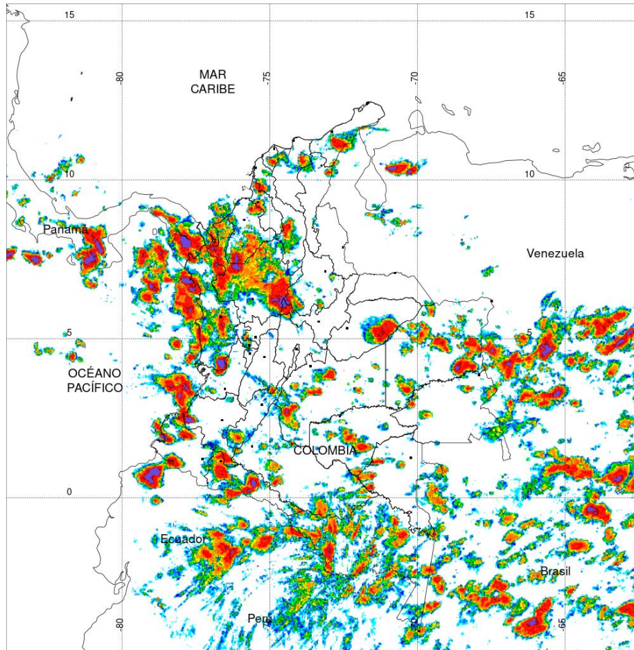
PRECIPITACIÓN TOTAL ACUMULADA POR ESTIMACIÓN SATELITAL (GOES-16) MAY 16 DE 2020 (7:00) - MAY 17 DE 2020 (7:00)
