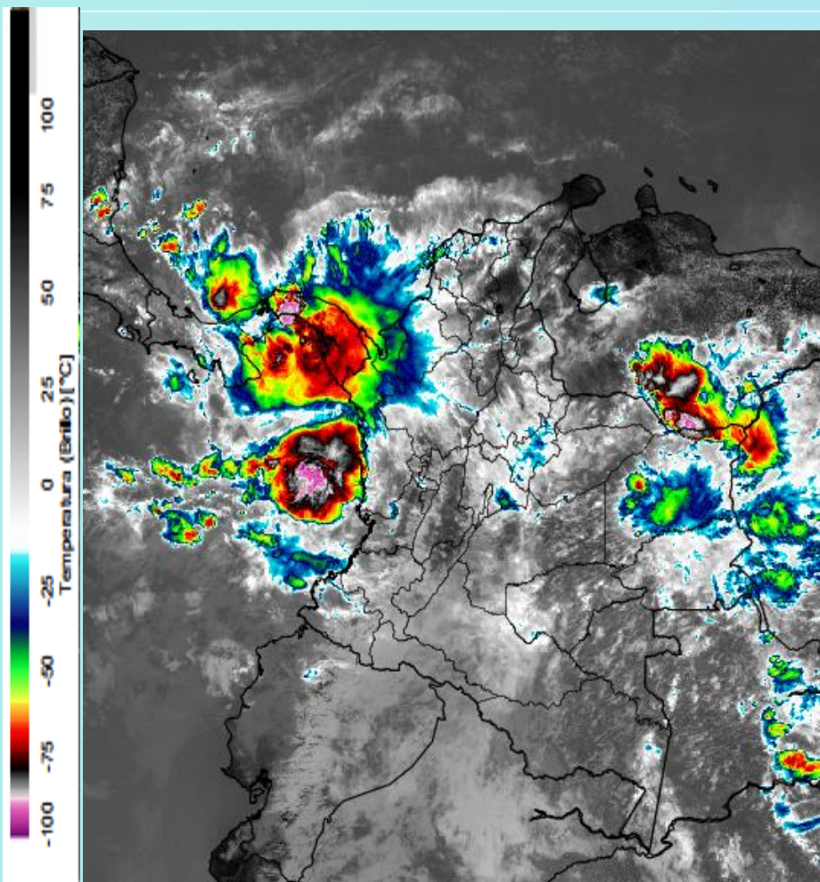
Imagen GOES East Canal Infrarrojo, 17 de mayo de 2020. Hora 12:00 HLC. Fuente: IDEAM-GOES 16
