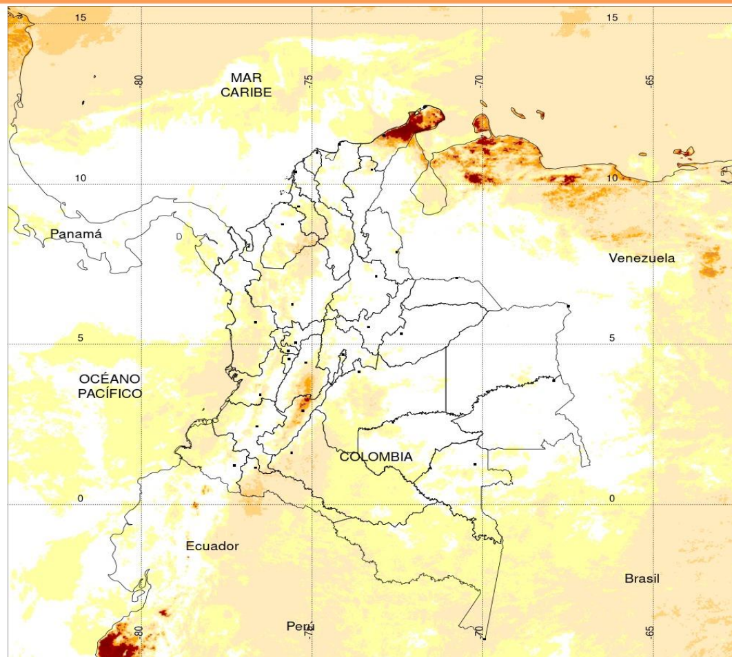
TEMPERATURA SUPERFICIAL MÁXIMA POR ESTIMACIÓN SATELITAL (GOES-16) ( 2020-07-11 09:00:00 a 2020-07-11 12:40:00 )
