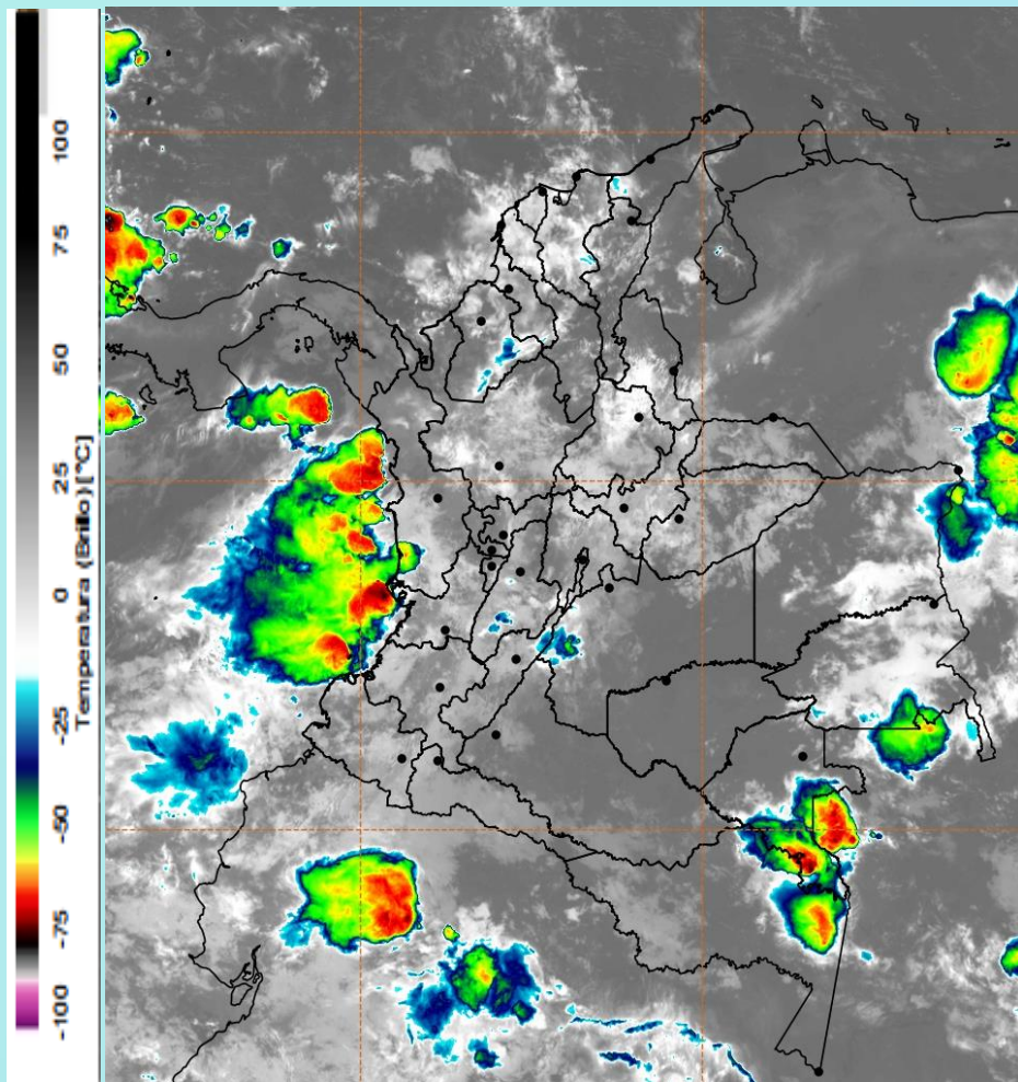
Imagen GOES East Canal Infrarrojo, 13 de julio de 2020. Hora 06:50 HLC. Fuente: IDEAM-GOES 167
