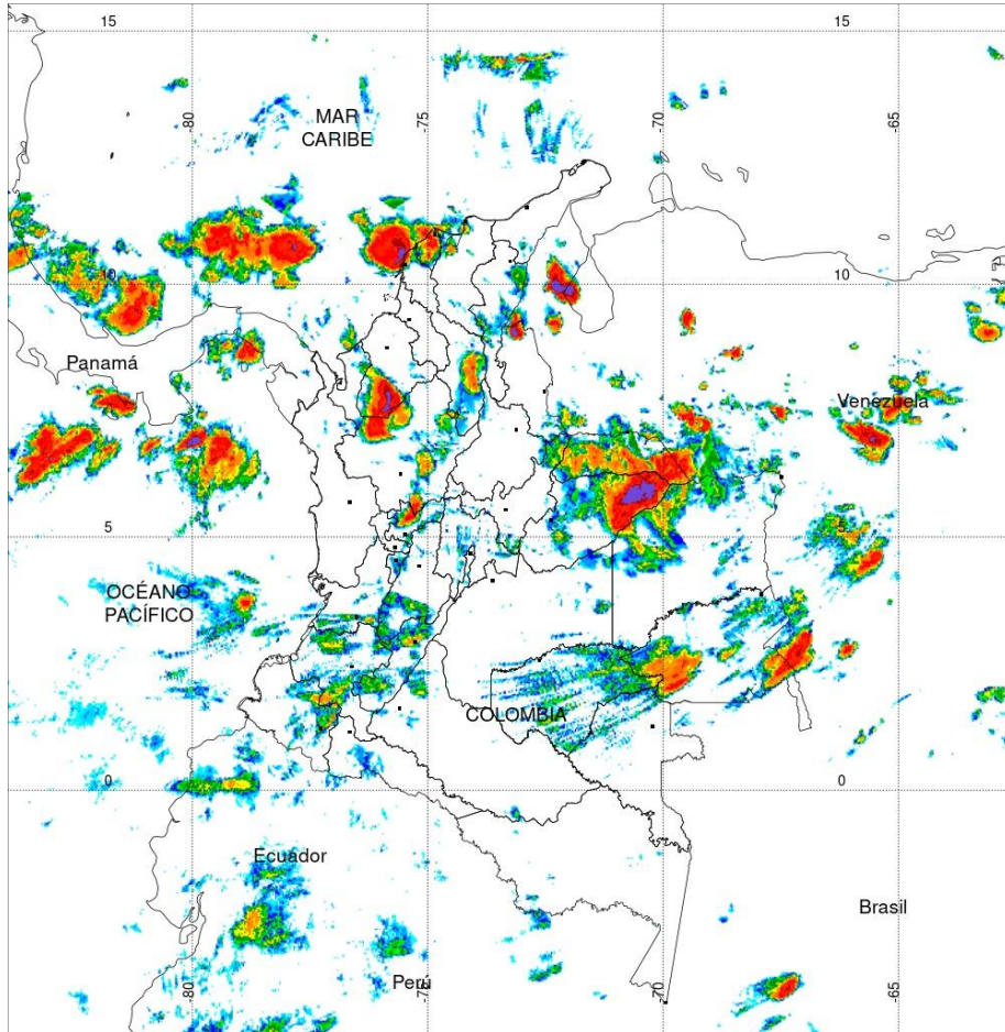
PRECIPITACIÓN TOTAL ACUMULADA POR ESTIMACIÓN SATELITAL (GOES-16) JUL 11 DE 2020 (7:00) - JUL 12 DE 2020 (7:00)
